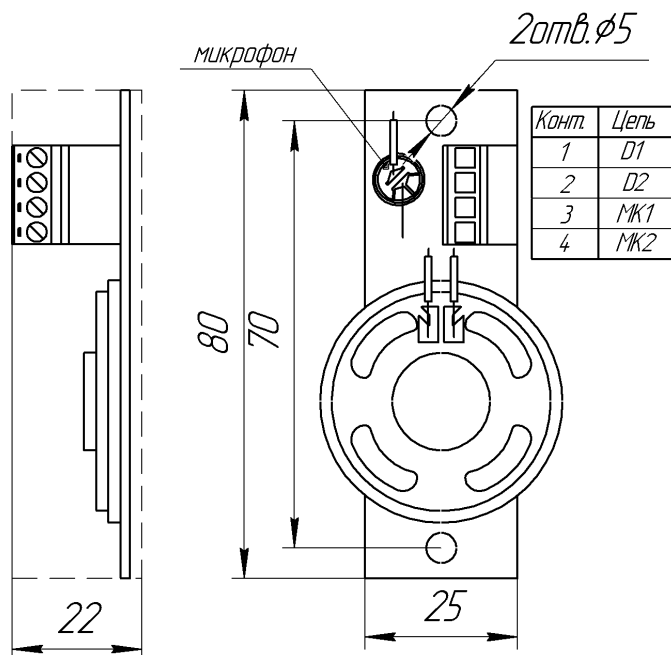
Рис.1. Габаритные, установочные размеры и назначение колодок
